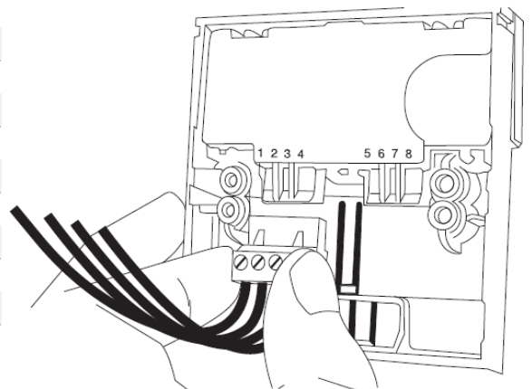
Присоединение при помощи съемных клемников
