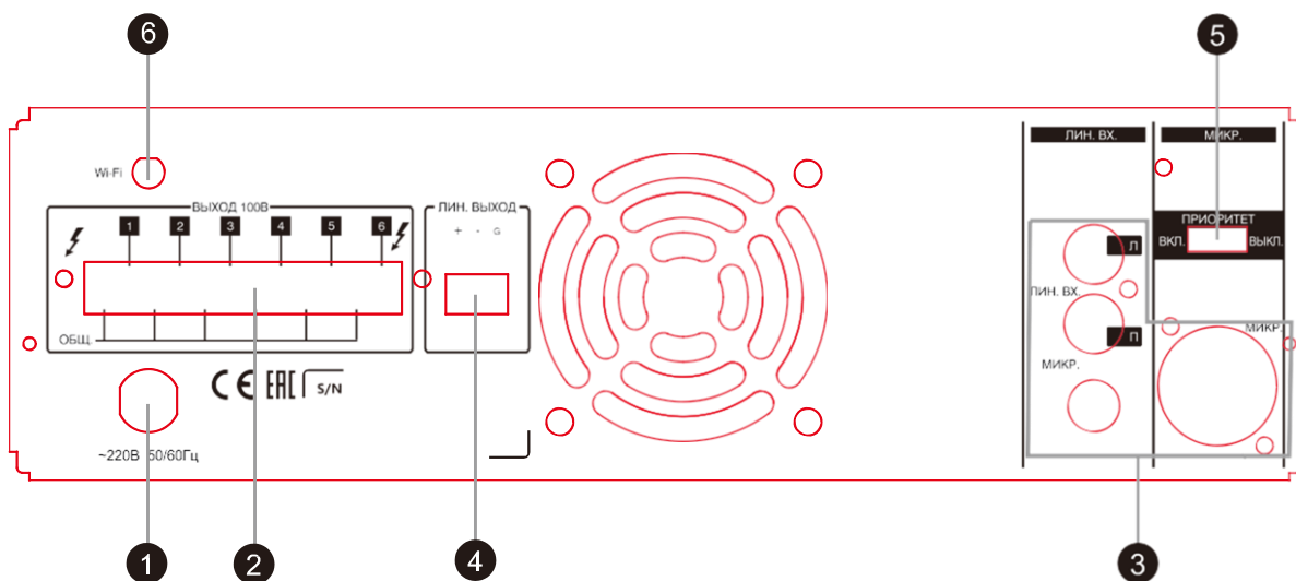
Рис. 3.2. Задняя панель LPA-DotCom
