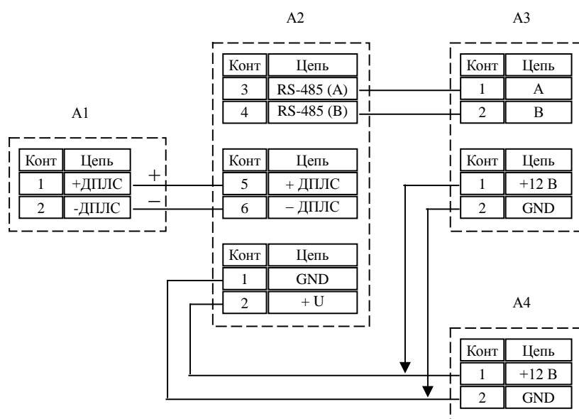
A1 – извещатель; A2 – «С2000-КДЛ»; A3 – пульт контроля и управления «С2000», «С2000М»; A4 – источник питания 12В
